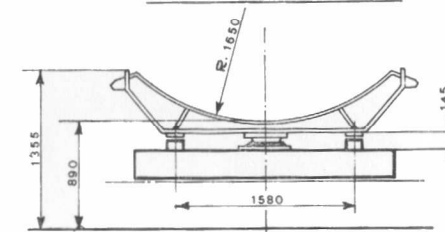
Sez. B-B scala 1:40
